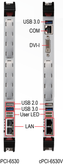
cPCI-6530
